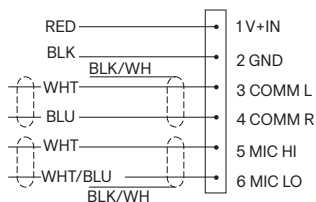
航空機インターフェイス構成図
